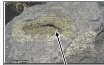
Figure 2 : Enclave du socle granitique dans une coulée de basalte
