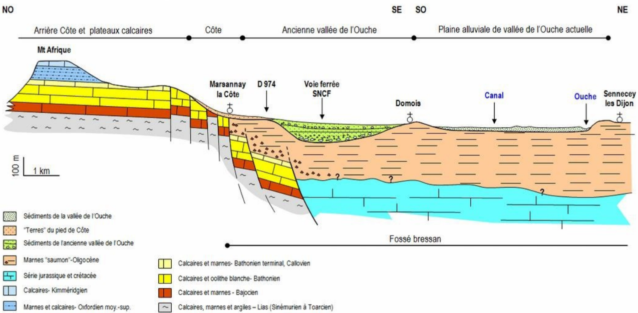
Fossé d'effondrement : au sud de Dijon, le fossé bressan, la Côte et le Mont Afrique Modifié d'après schéma page 20 du fascicule « Journée d'étude sur l'eau. 28-02-1990- conseil général de Côte d'Or »
