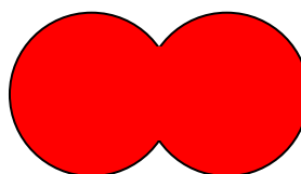
Dioxygène : O 2
