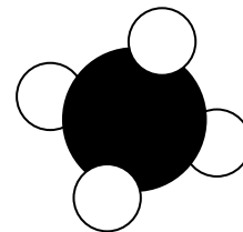
Méthane : CH 4
