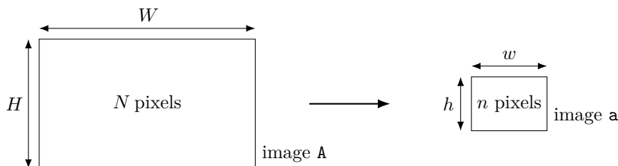
Figure 3 Redimensionnement d'image
