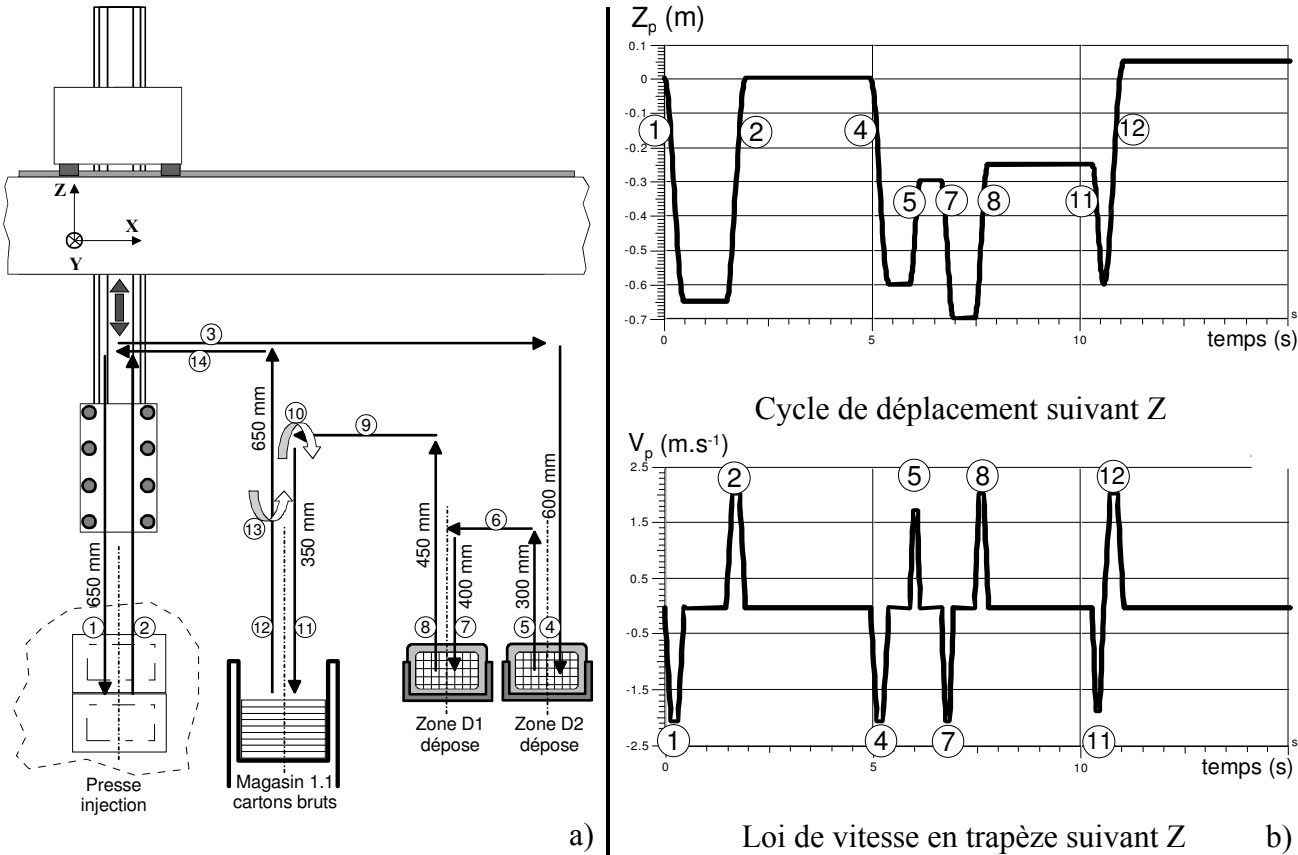
Figure 1.3 : a) Cycle étudié pour l'axe Z – b) Loi de mouvement pour l'axe Z
