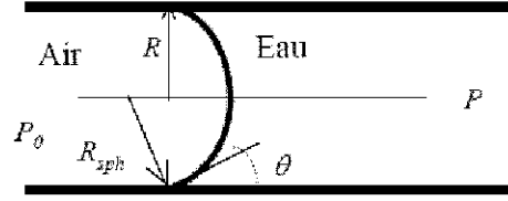
FIG. 15 – Pore cylindrique.
