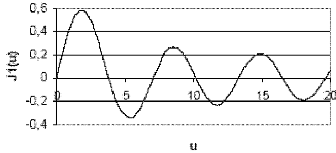
FIG. 7 – Graphe de la fonction de Bessel J_1(u)
