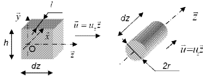
FIG. 10 – Eléments de volume soumis à une force de viscosité en coordonnées cartésiennes et en coordonnées cylindriques.
