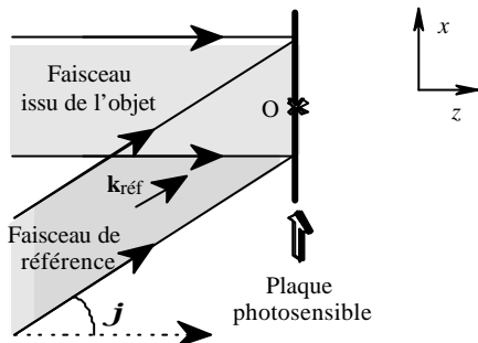
Fig. 1 Enregistrement d'un hologramme mince
