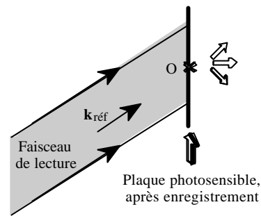
Fig. 2 Lecture en transmission d'un hologramme mince
