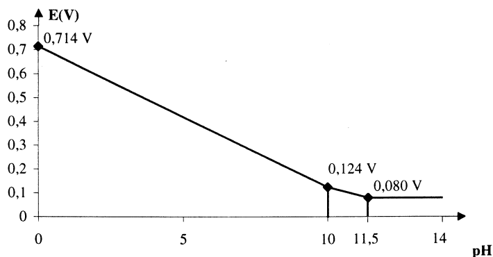
Figure I - Diagramme potentiel normal apparent-pH du révélateur
