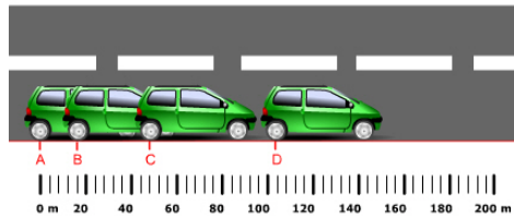
حركة متسارعة
