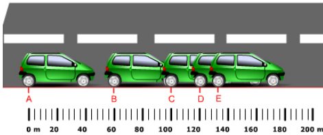
حركة متباطئة
