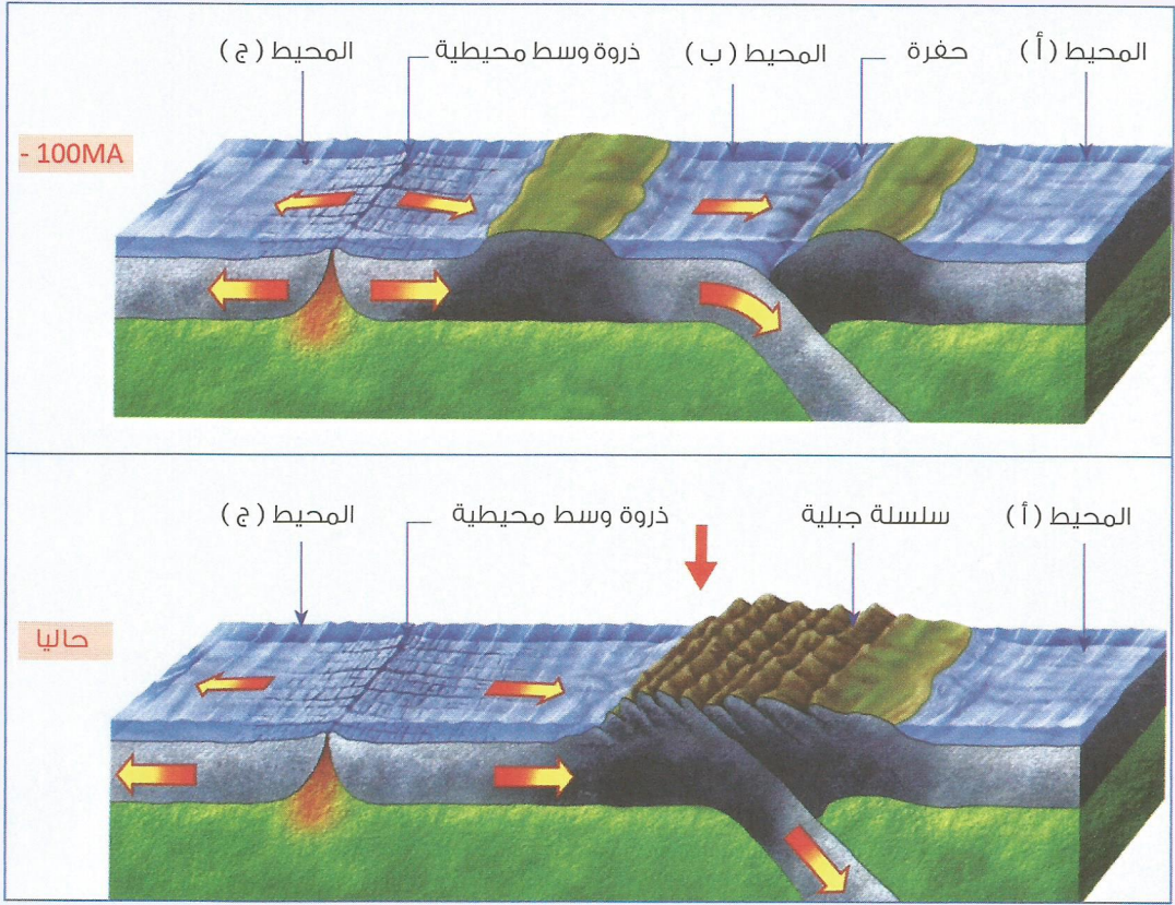
وث. سلاسل الطمر – Chaîne de subduction
