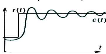
Système stable mal amorti
