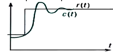
Système stable bien amorti
